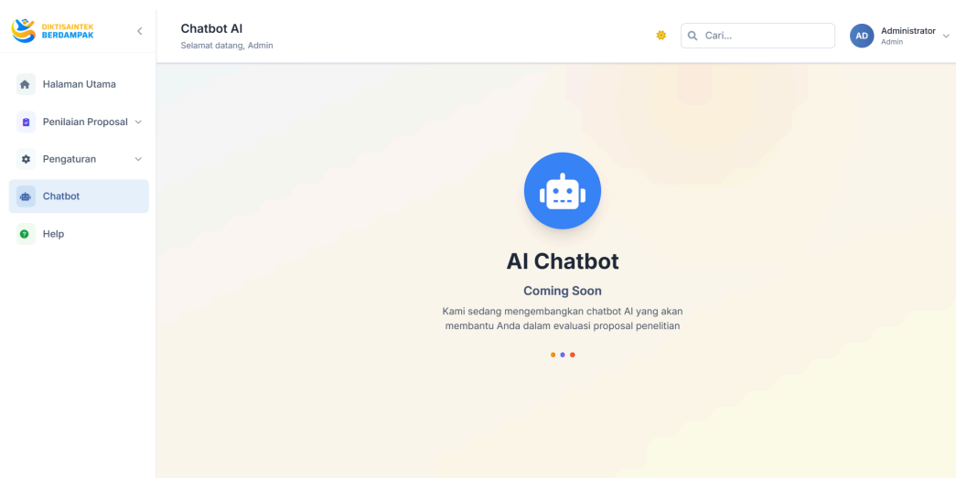
Gambar 26. Chatbot
