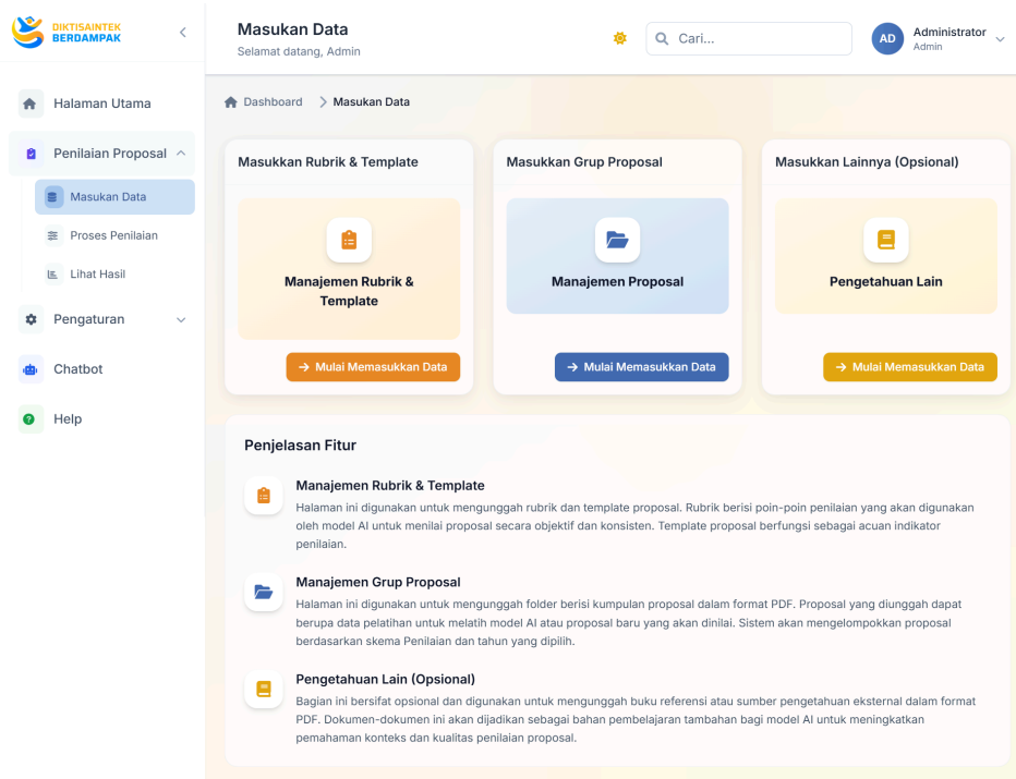
Gambar 8. Masukan Data
