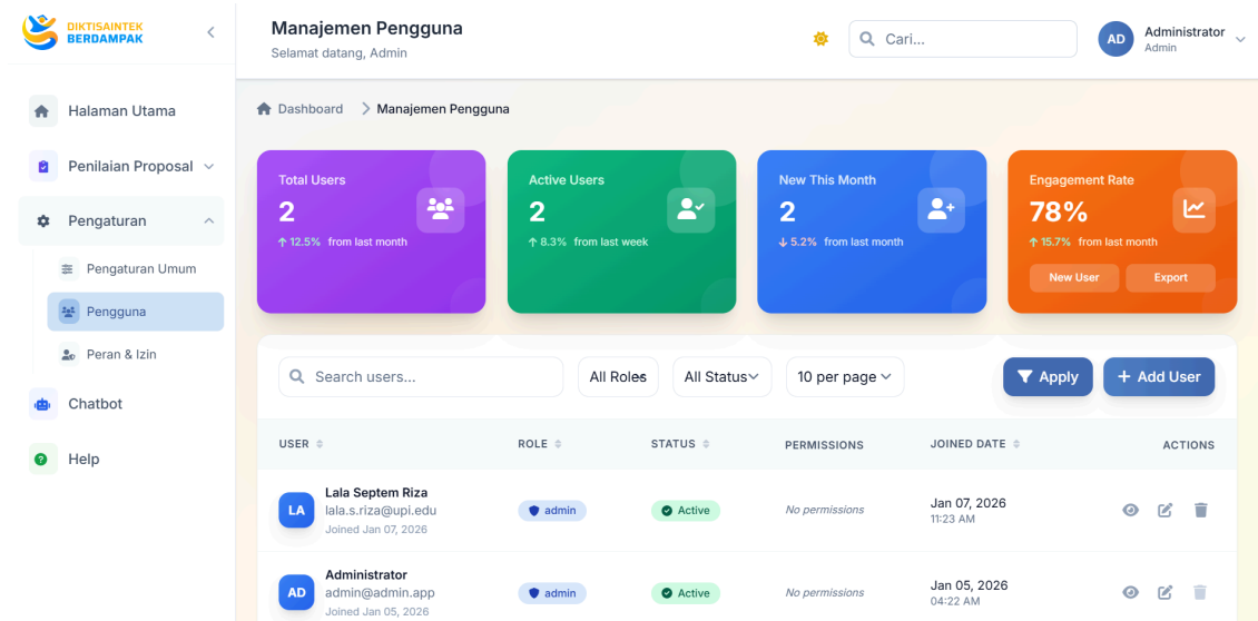
Gambar 23. Manajemen Pengguna
