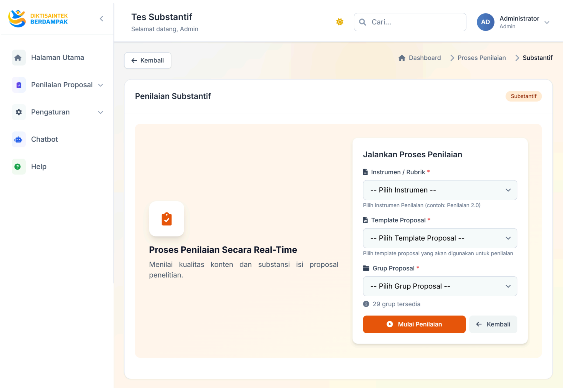
Gambar 15. Tes Substantif
