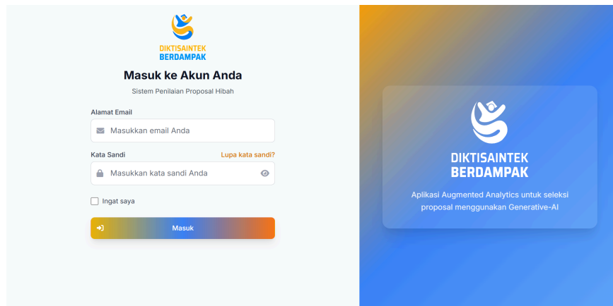
Gambar 5. Login
