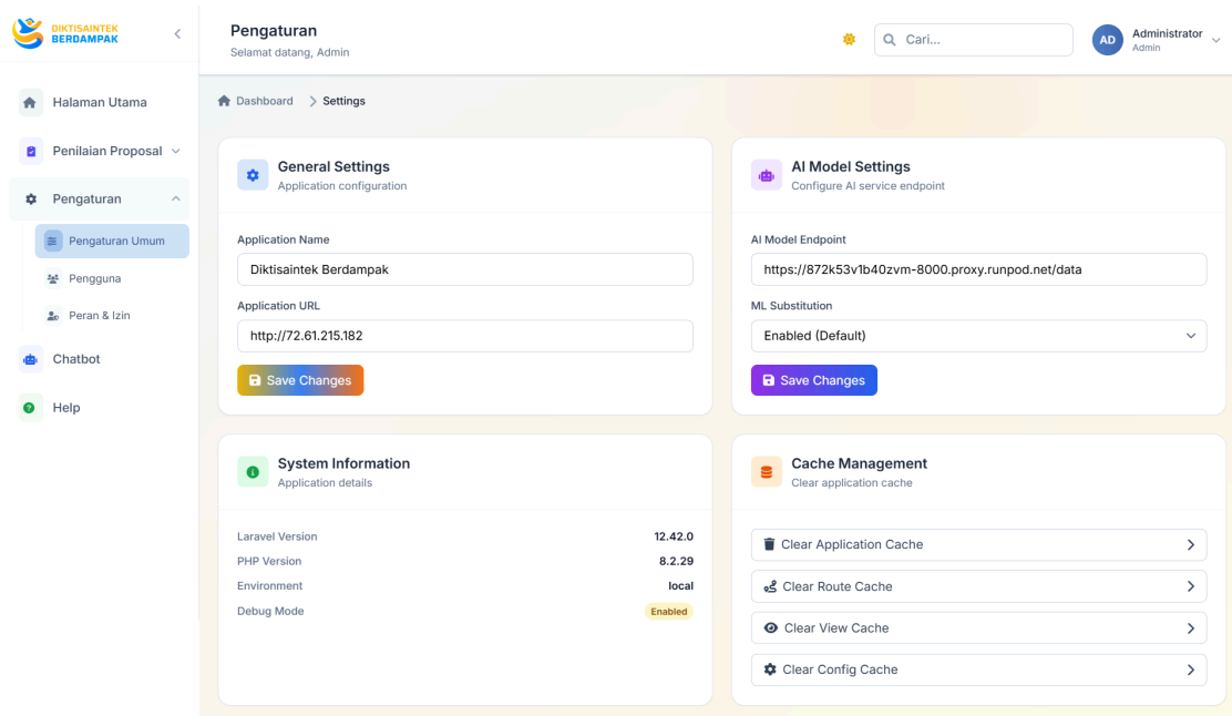
Gambar 22. Pengaturan Umum
