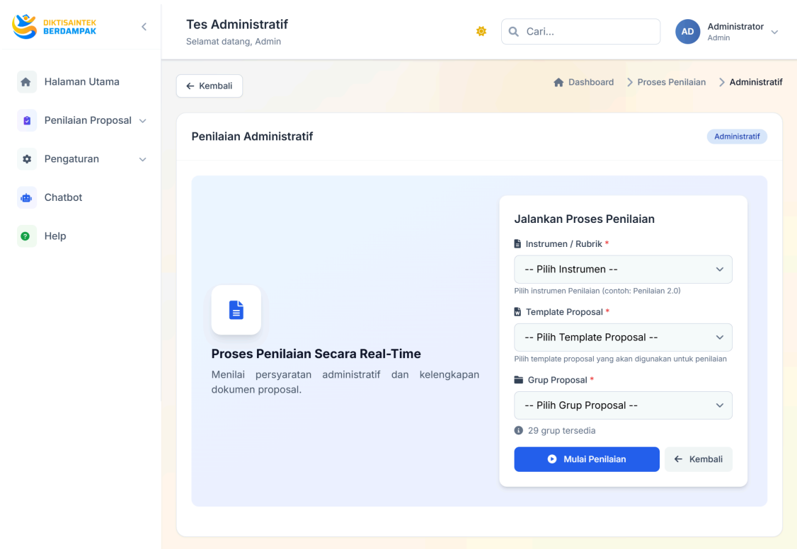
Gambar 14. Tes Administratif
